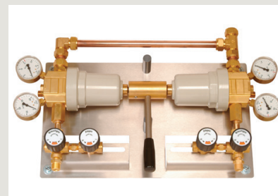
Bild 1, semiautomatisk tömningscentral
